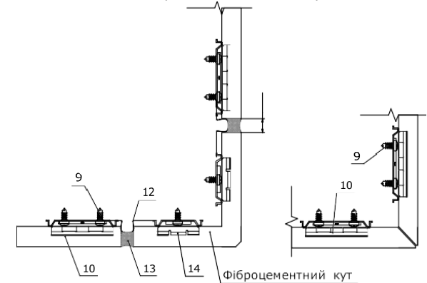
Варіанти виконання кута
